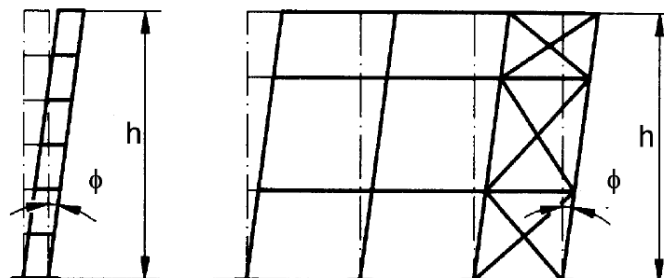
Figura C4.2.2 Imperfezioni globali equivalenti
