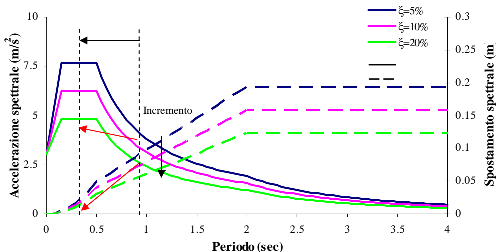
Figura C7A.10.1 - Strategie di riduzione della domanda mediante dissipazione di energia
